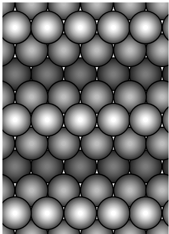
Pt(110)(1x2)
