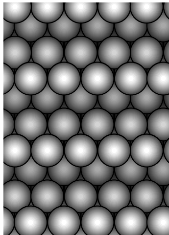
Pt(331)
