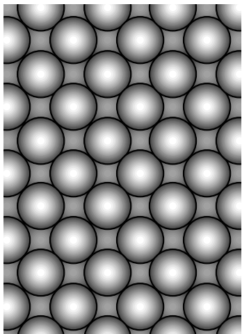
Pt(100)(1x1)
