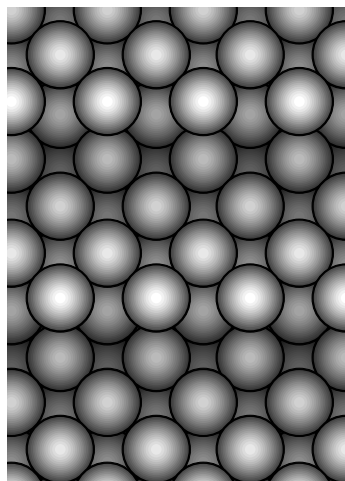
Pt(410)
