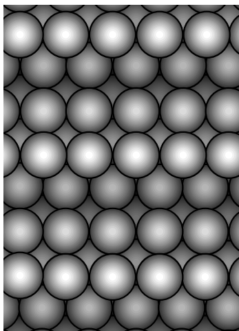
Pt(511)
