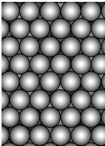
hex-Pt(100)
