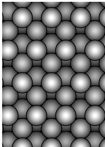
Pt(210)
