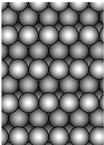
Pt(331)
