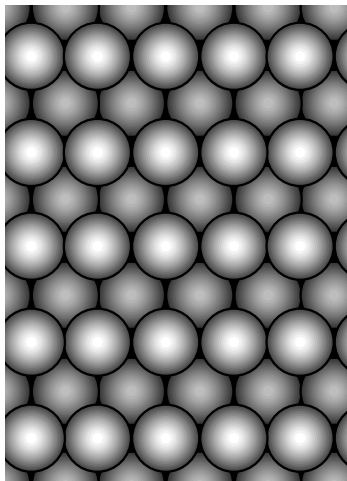
Pt(110)(1x1)
