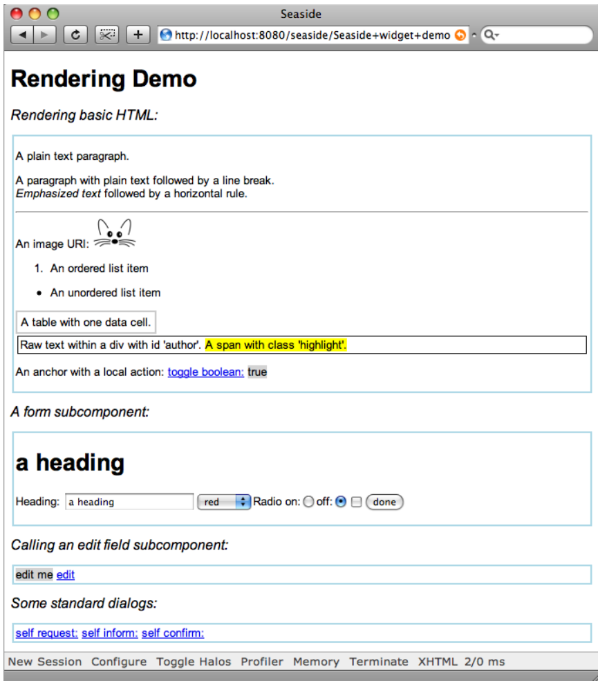
Figure 13-13 RenderingDemo.
